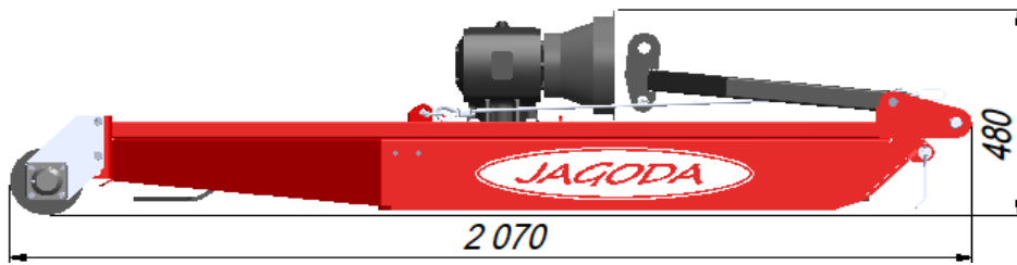
ВИД сбоку
