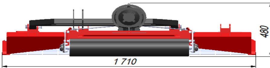
ВИД сзади
