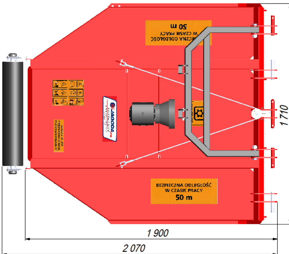
ВИД сверху
